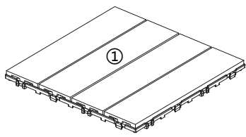
400x400x23mm x49
