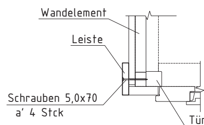
Konstruktion Zeichnung-4
