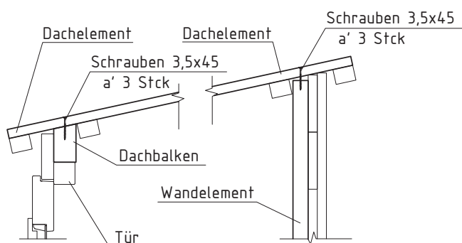
Schnitt 3-3
