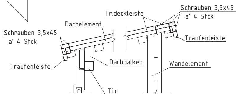
Schnitt 5-5
