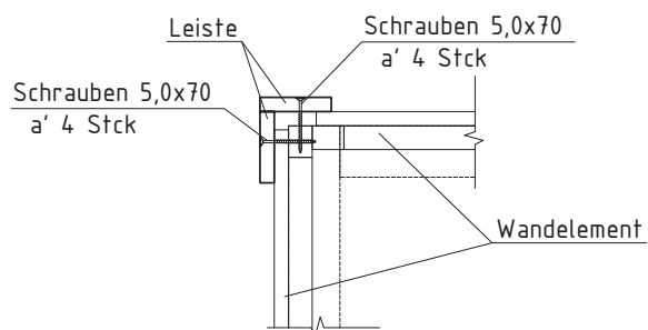
Konstruktion Zeichnung-3
