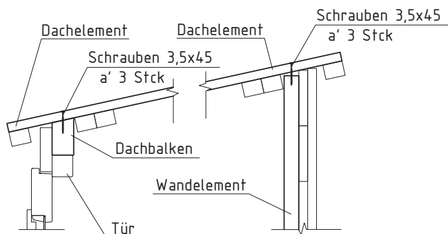
Schnitt 5-5
