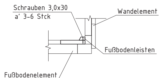
Schnitt 6-6
