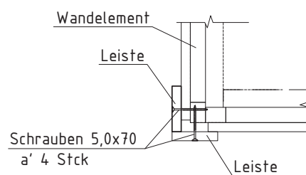
Konstruktion Zeichnung-5
