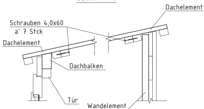
Schnitt 4-4
