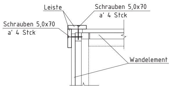
Konstruktion Zeichnung-4
